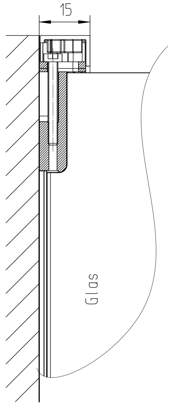
Schnitt A-A
